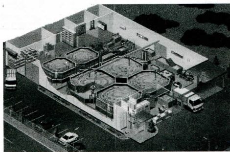
圖 11-13 室內循環水養殖系統之示意圖
